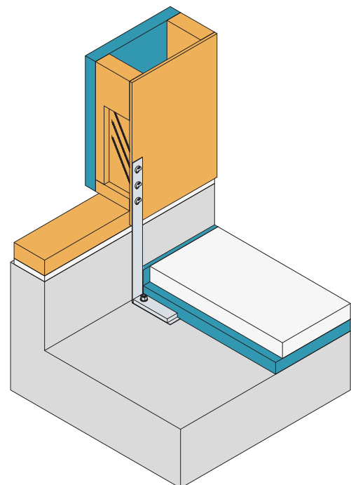
Anschluss an Holzrahmenwände
