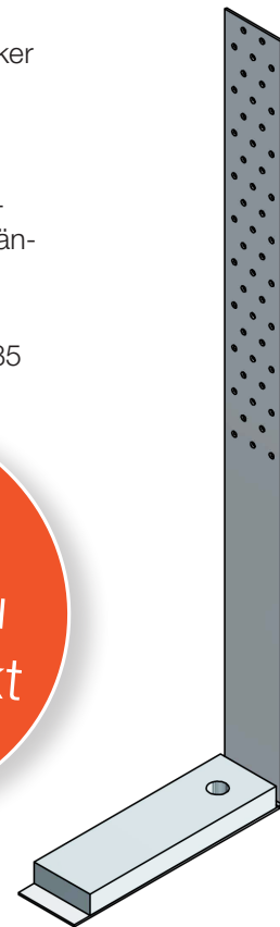
Zuganker HD mit Sonder-Lochbild
