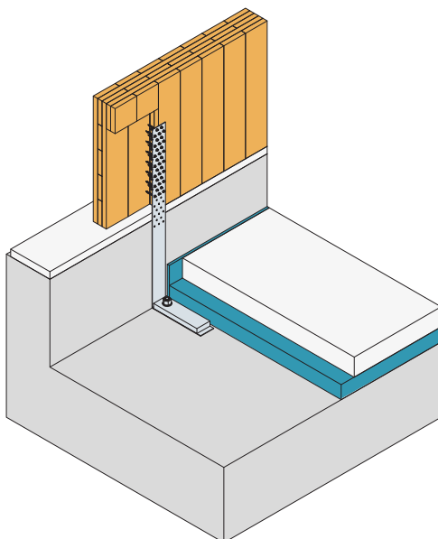
Anschluss an Brettspertholzwände
