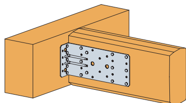
ABR220 Nebenträger an Hauptträger
