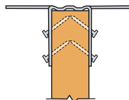
LSSU Nägeln im Nebenträger
