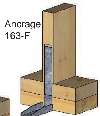
Partie inférieure courte
