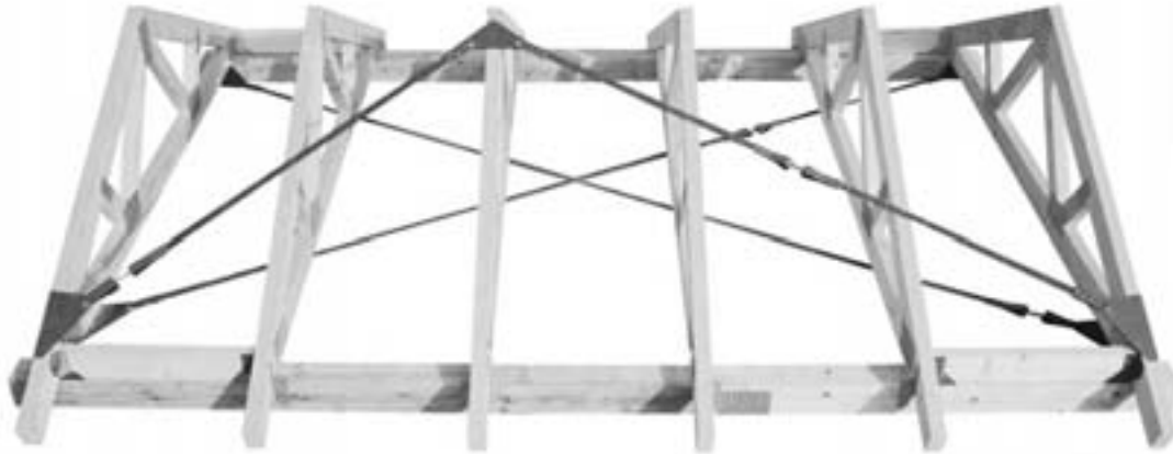
Windaussteifung einer Dachfläche mit Bandanschluss K25 am Firstpunkt und Bandanschluss F25 am Sparrenfuß.
