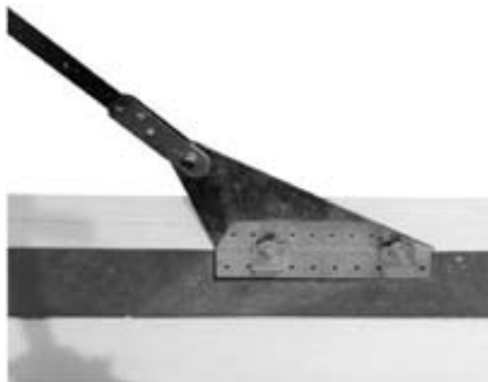
Detail am Fundament: Bandanschluss G25 auf Beton verbolzt. Lastverteilung durch die BMF U-Scheibe 40 × 50 × 10.
