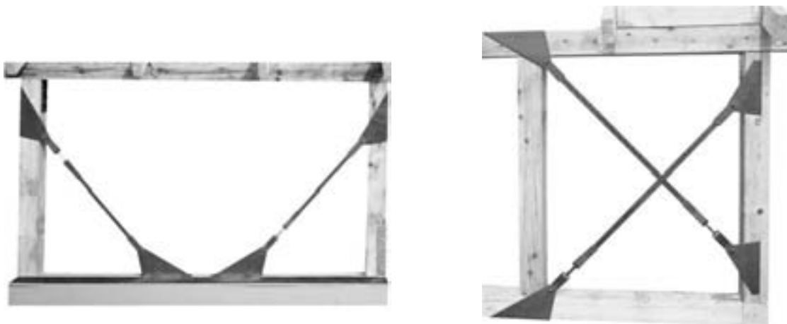
Wandaussteifung mit Bandanschluss F25 oder G25 an einer Eckstütze. Und mit G25 an einem Betonfundament.
