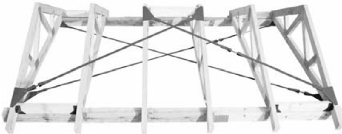
Windaussteifung einer Dachfläche mit Bandanschluss F25 oder G25 am Firstpunkt und am Sparrenfuß.
